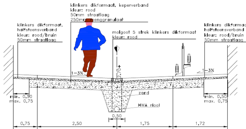
Profiel D-D
