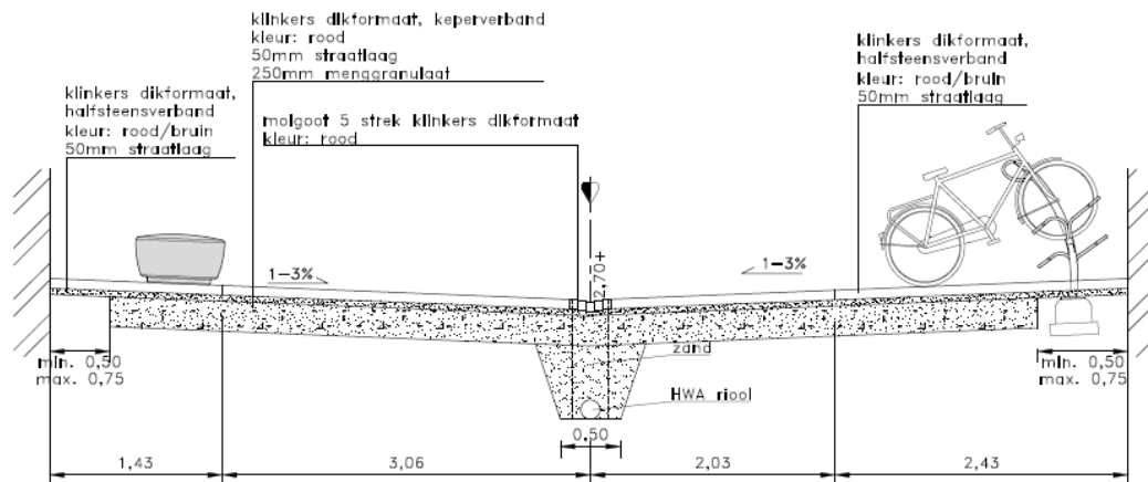
Profiel C-C
